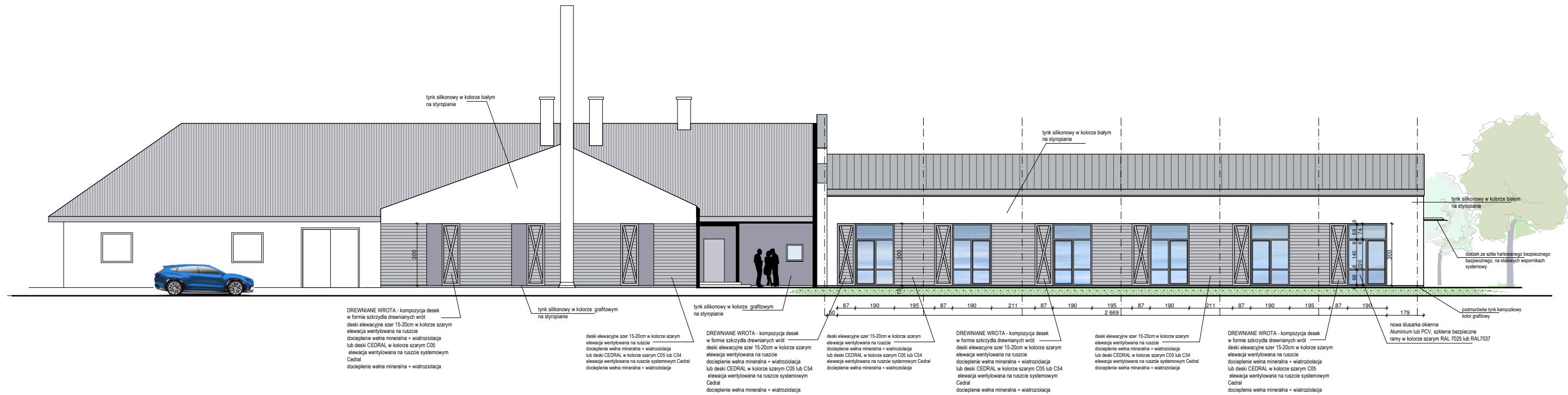
PROJEKT TERMOMODERNIZACJI UJEŹDŹALNI ELEWACJA BOCZNA1 WARIANT 1
